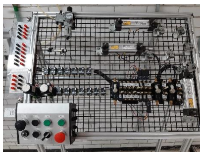
Mesa neumática
